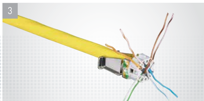
Разделить проводники и зафиксировать на позициях, показанных на рисунке
