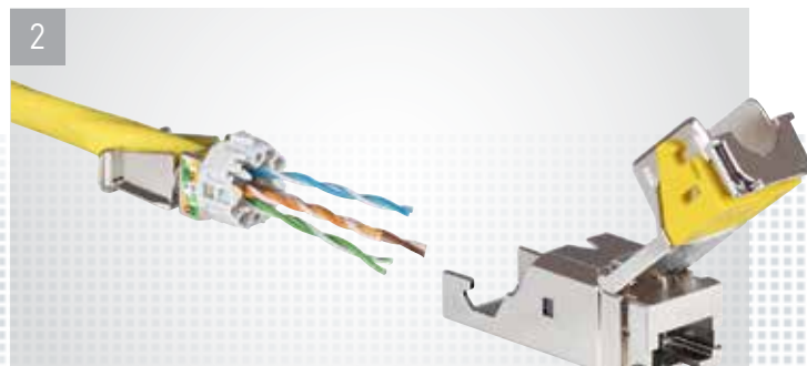
Пропустить пары кабеля сзади через основание коннектора
